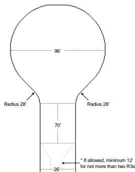
96 Foot Cul-de-sac
