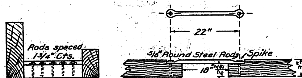
Section C-D
