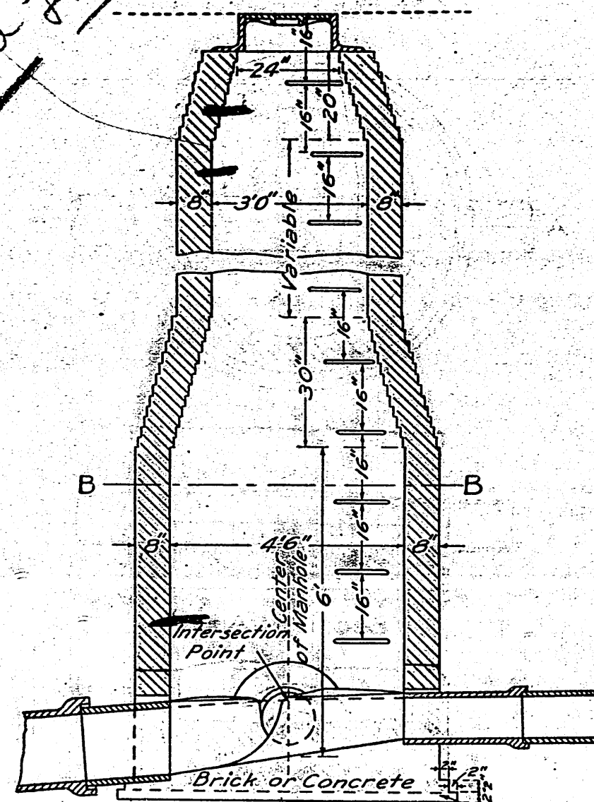
Section A-A
