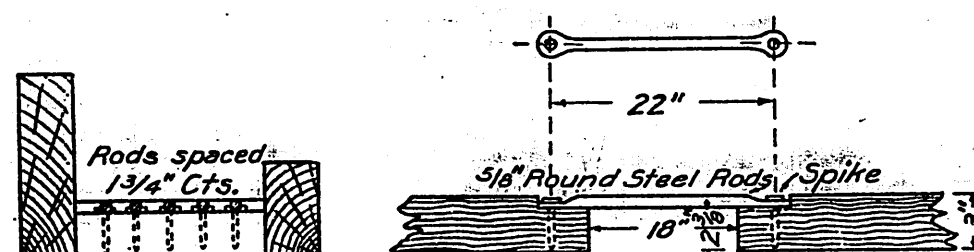
Section C-D
