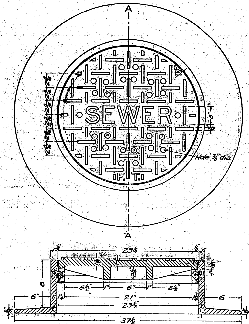
Section A-A
